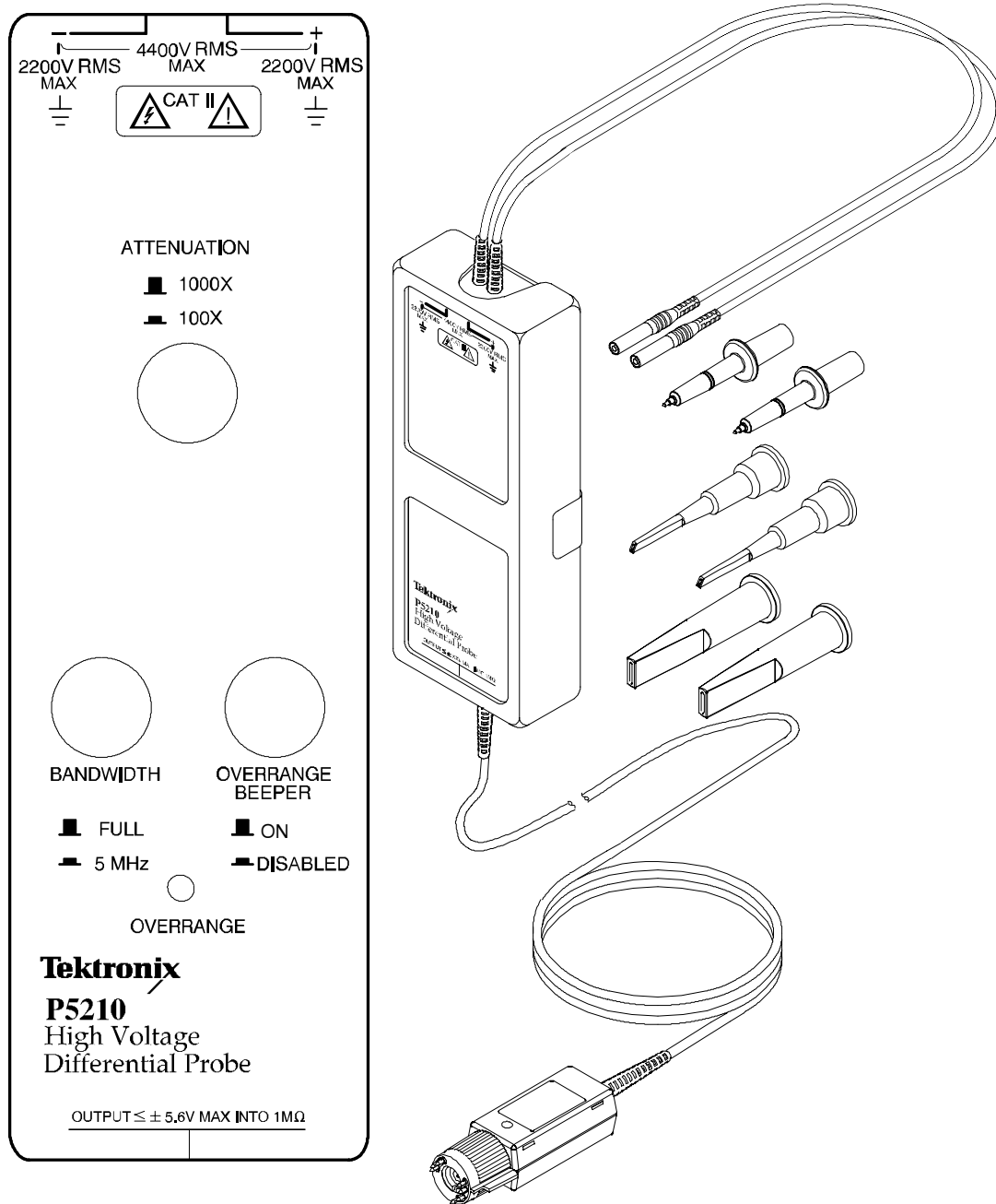
Abbildung 1: P5210 Hochspannungs-Differentialastkopf
