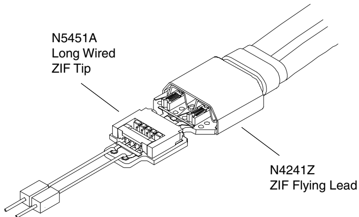
Figure 59 N5451A Long Wired ZIF Tip
