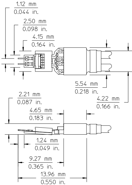
Figure 58 N5426A ZIF Tip Dimensions
