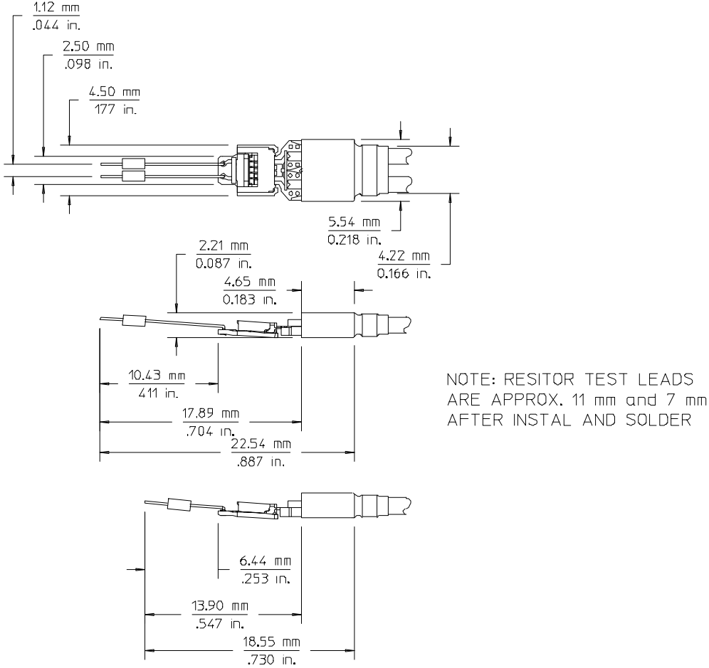
Figure 60 N5451A Long Wired ZIF Tip Dimensions
