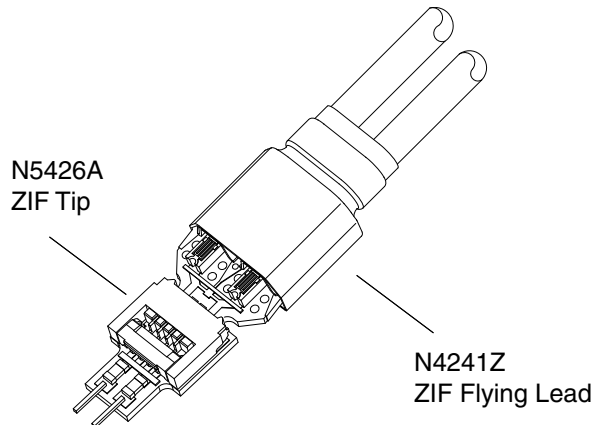
Figure 57 N5426A ZIF Tip
