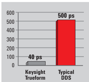
Jitter
